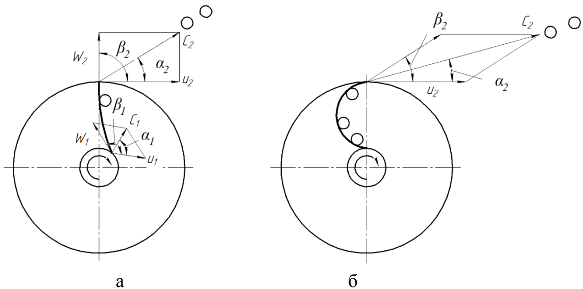
Рис. 1. Схема руху частинок льоду при криогенному бластингу а – радіальне розташування направляючих жолобів ( \beta_1=90^\circ ); б – жолоби загнуті вперед у напрямку обертання ( \beta_1<90^\circ );
