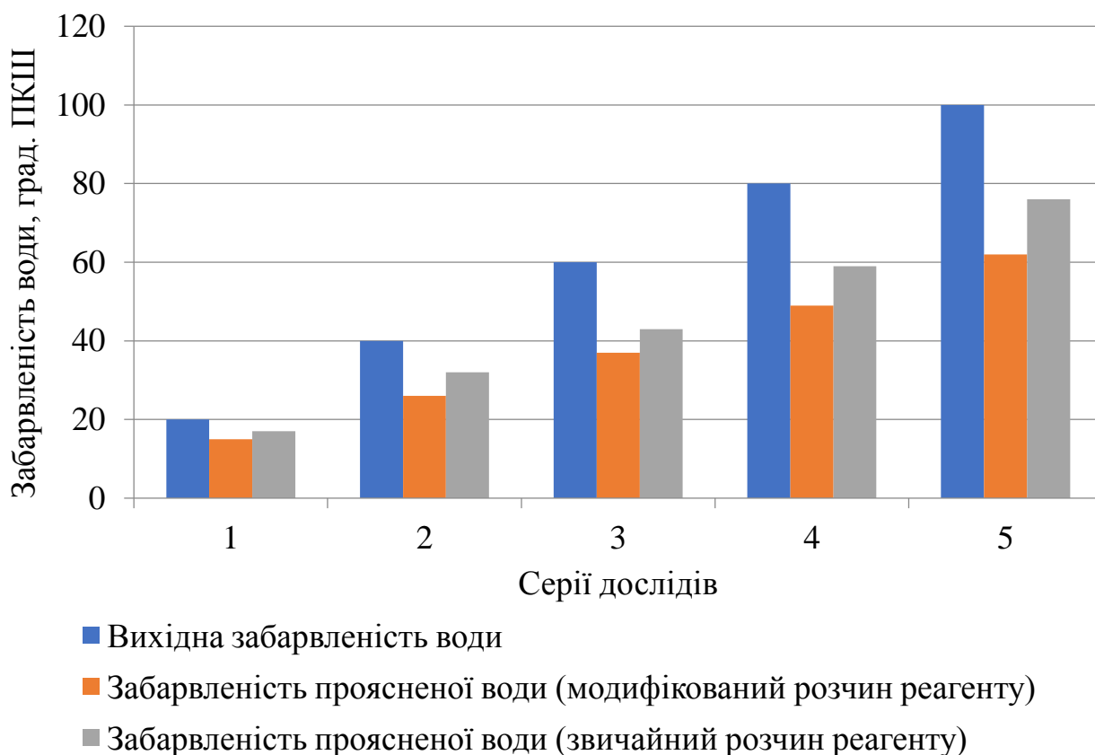
Рис. 1. Вплив модифікованого розчину коагулянту сульфату алюмінію на знебарвлення маломутних забарвлених вод
