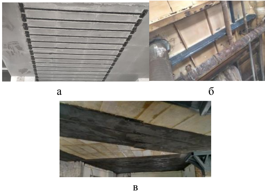
Рис. 1. Підсилення конструкцій зовнішнім армуванням: а – плити перекриття ламелями; б – ребристої плити; в – плити перекриття волокном
