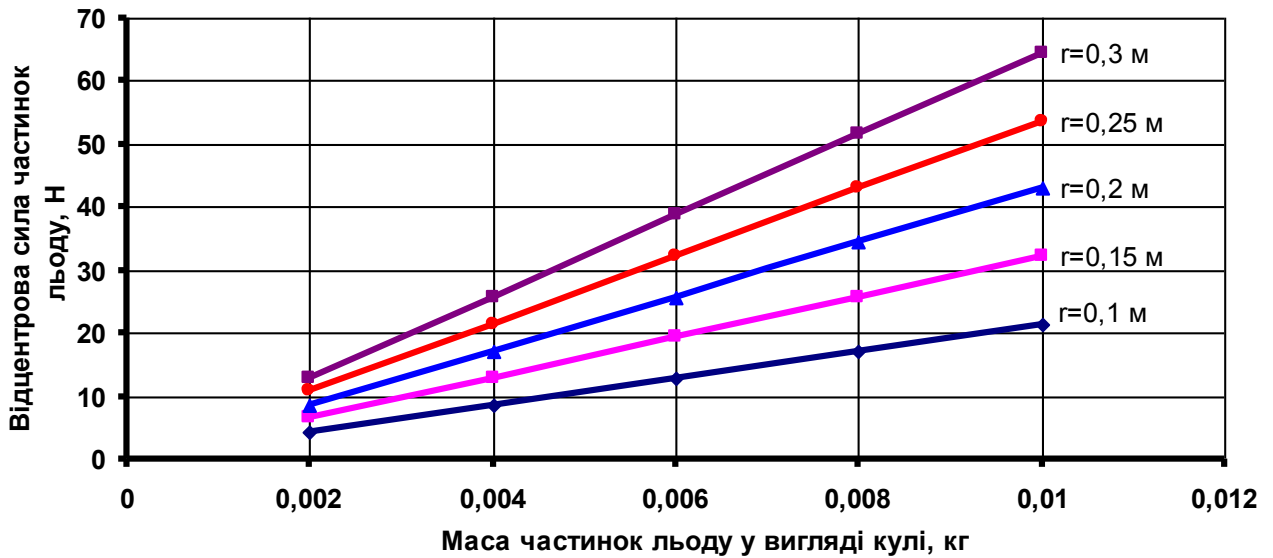
Рис. 2. Залежність відцентрової сили частинок льоду від маси кулі при 1400 оборотів диска в хвилину
