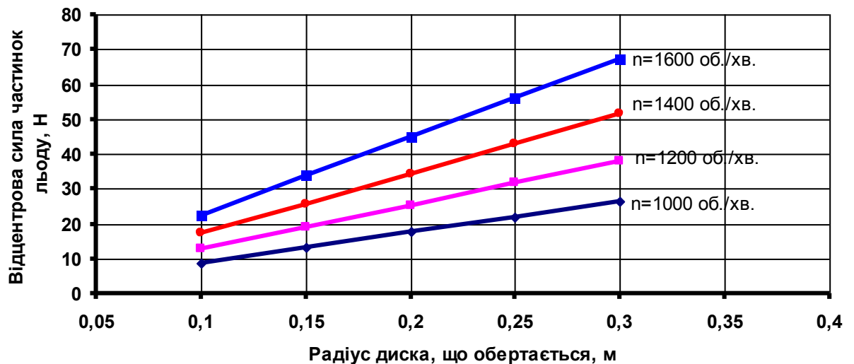
Рис. 3. Залежність відцентрової сили частинок льоду від радіуса диска, що обертається, при масі кулі 0,008 кг
