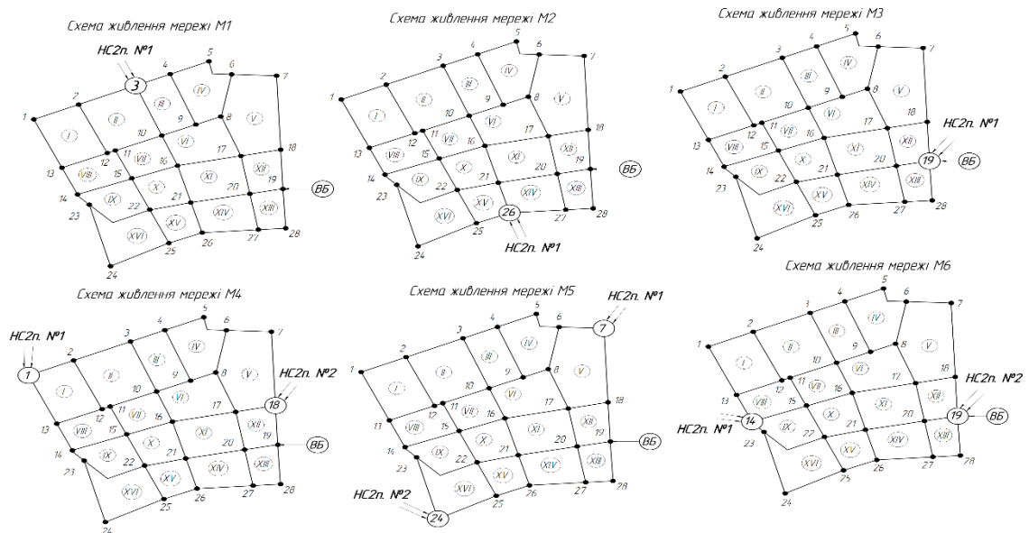
Рис.1. Моделювання варіантів живлення водопровідної мережі
